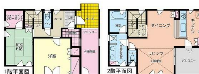
間取図 (平面図)
