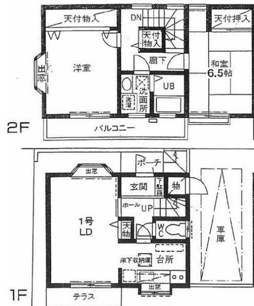
間取図 (平面図)
