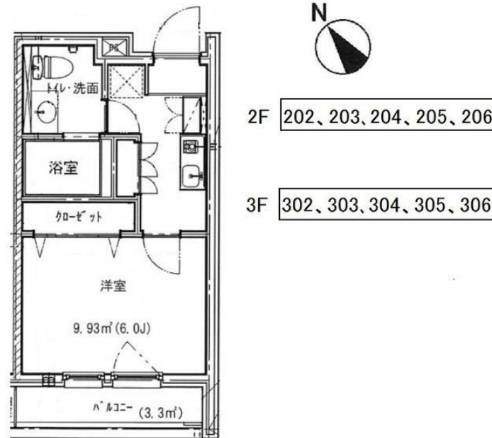
間取図 (平面図)
